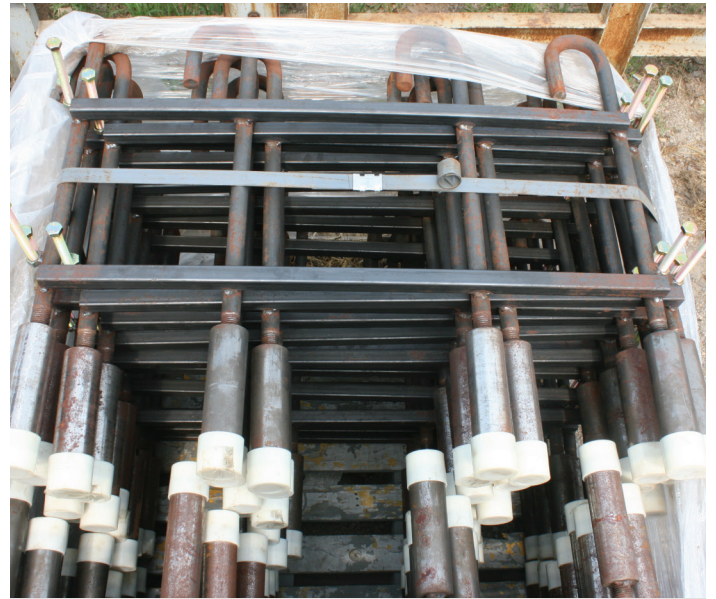
옹벽용 J 양카SET
