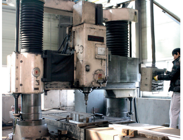
플라노밀러 1200x2000
