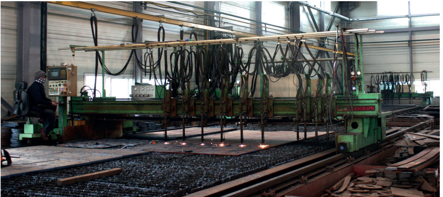
대형 CNC모형절단기 6000x15000 1대
