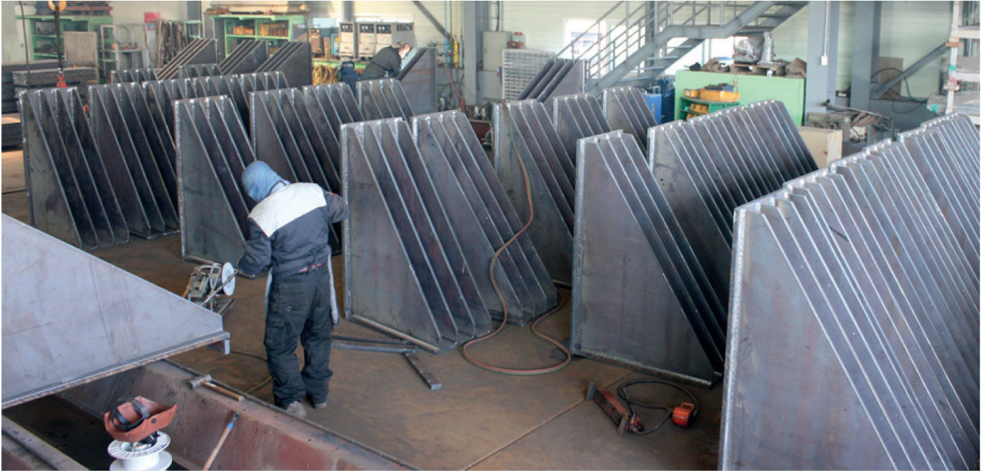
고속철도 내진 보강 브라켓트
